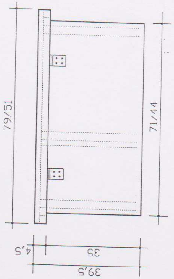
Seitenansicht A/C
